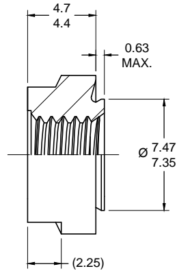
SECTION A-A SCALE 3:1
